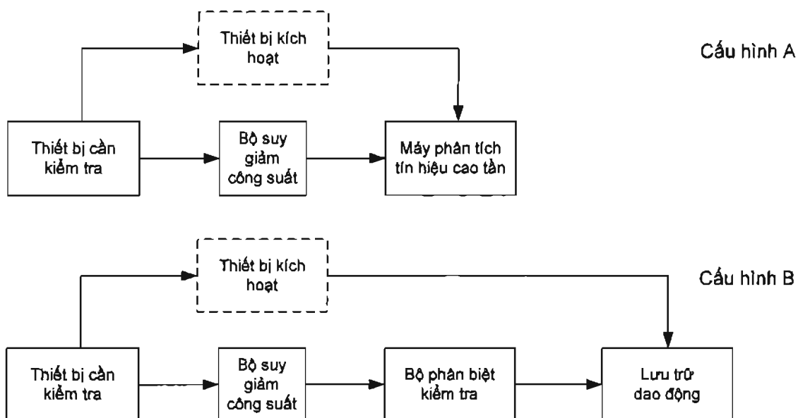
Hình 5 - Phép đo độ chính xác điều chế
