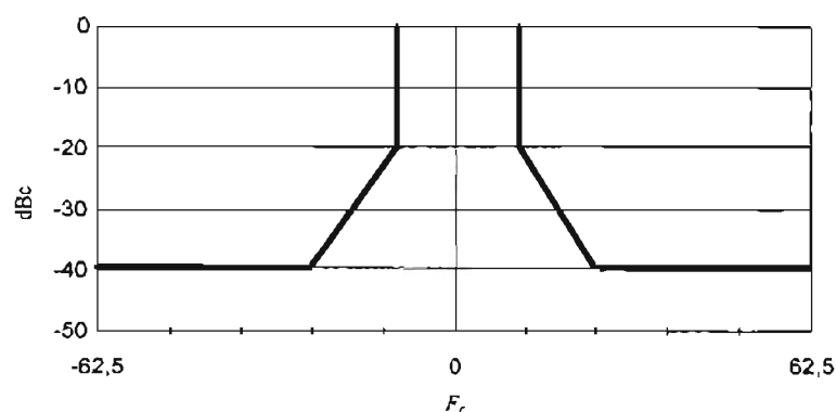
Hình 4 - Mặt nạ phát xạ
