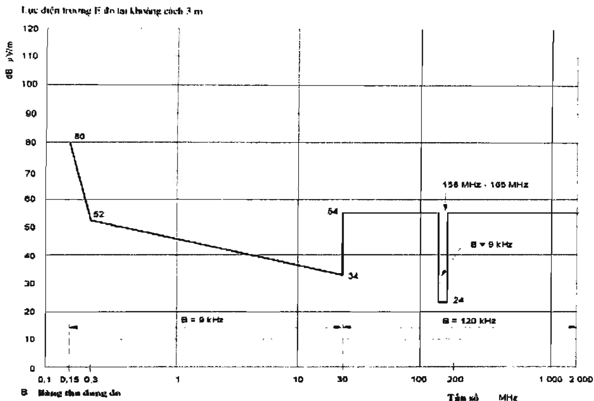
Hình 2 - Giới hạn phát xạ bức xạ từ các cổng vỏ
