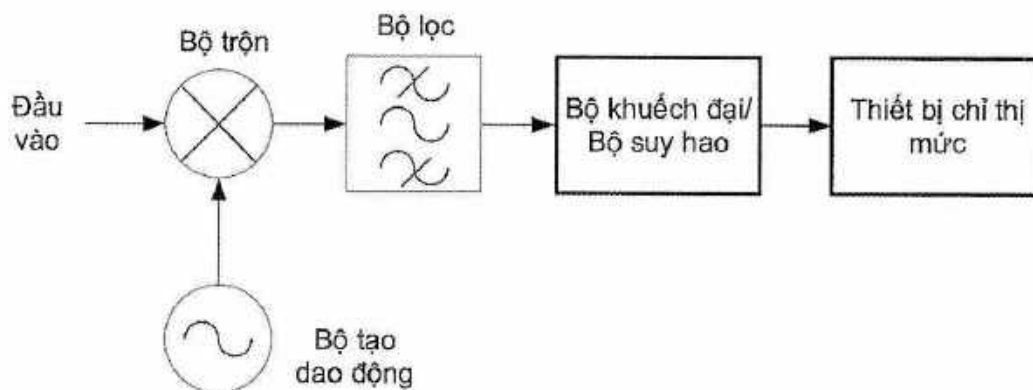
Hình A.1 - Máy thu đo công suất
