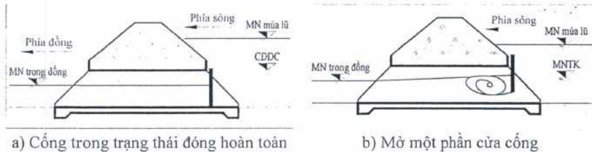
Hình 2. Sơ đồ vận hành cống tưới, cấp nước tự chảy trong mùa lũ.
