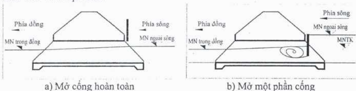
Hình 1. Sơ đồ vận hành cống tưới, cấp nước tự chảy trong mùa kiệt.
